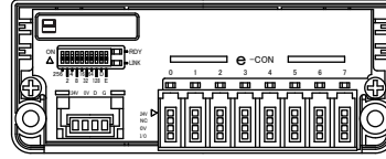
A. 出力用コネクタ (e-con スリーエムジャパン製)
