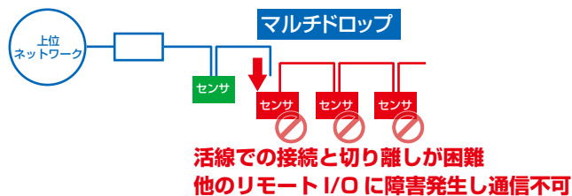
従来リモート I/O 通信方式
